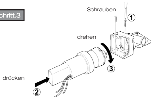
Abb 2. Die Pumpe darf nicht direkt an den Rumpf geschraubt werden
