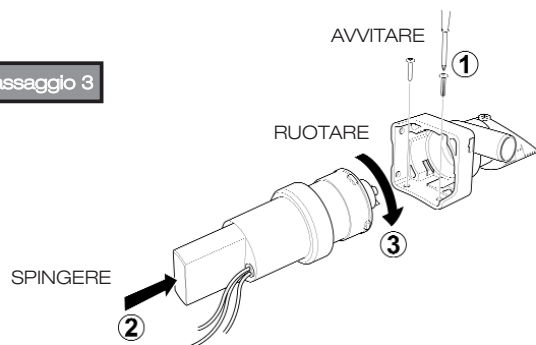
Figura 2 NON avvitare direttamente allo scafo
